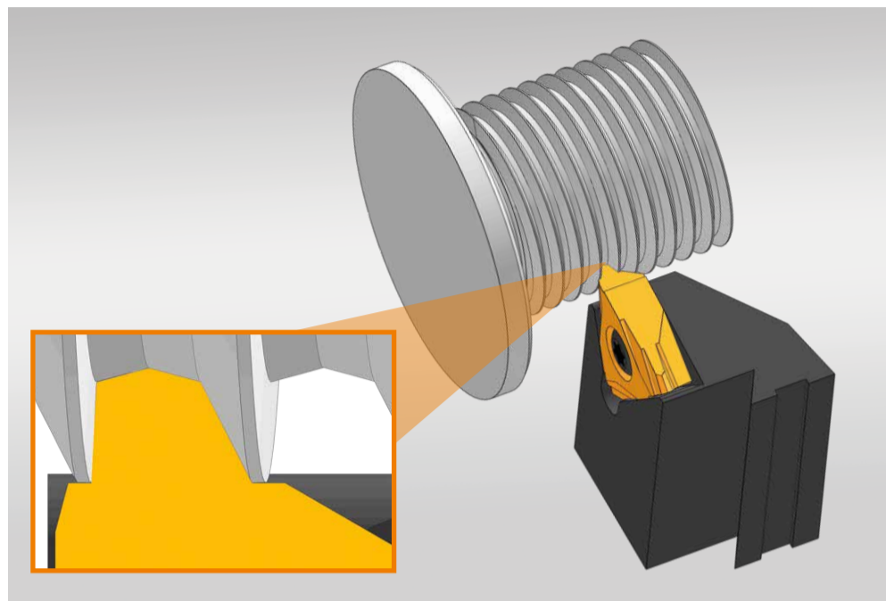
Esecuzione della filettatura monotagliente per filettature speciali
