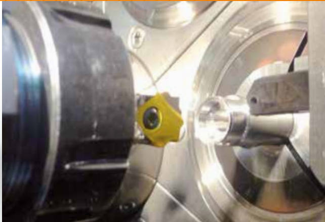
Wiertła kształtowe z płytkami wymiennymi
