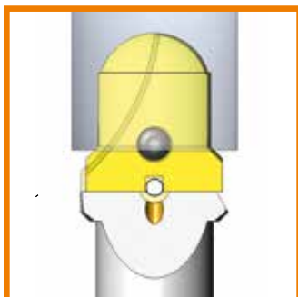
Wiercenie promienia płytką PWP
