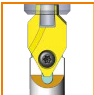
Wykonanie kanałka czołowego płytką PWP
