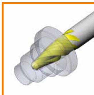
Wiercenie stożka wiertłem kształtowym krętym
