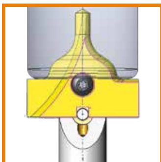
Wiercenie kształtowe w mosiądzu płytką PWP-D (Ustnik trąbki)
