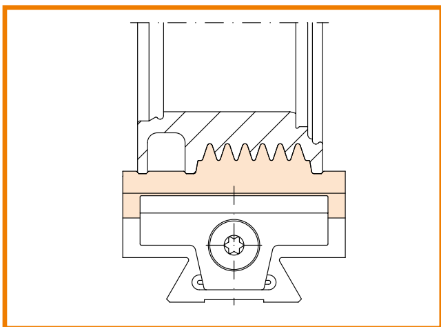
Sistema PWP-B
