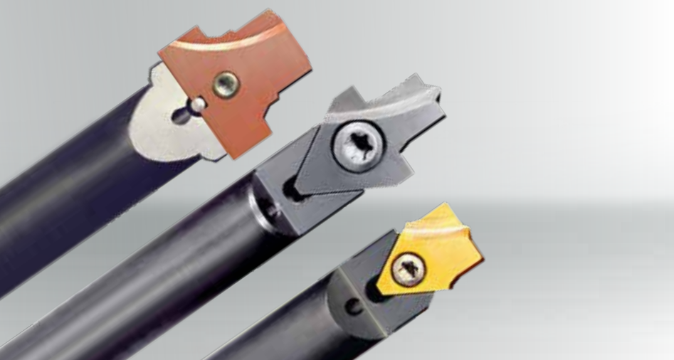
Perçage de forme avec plaquette interchangeable
