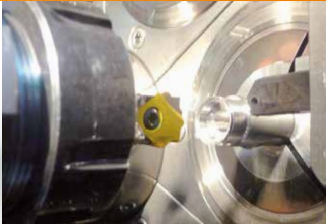
Perçage de forme avec plaquette interchangeable
