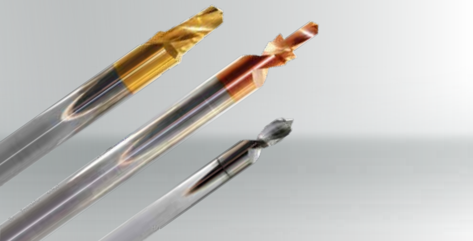
Perceur de forme carbure monobloc
