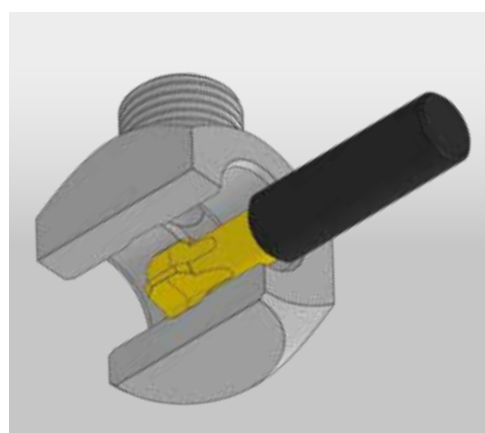
Lavorazione del contorno interno con fresa di forma Schwanog
