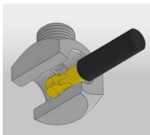
Tronzado interior con el fresado de forma de Schwanog
