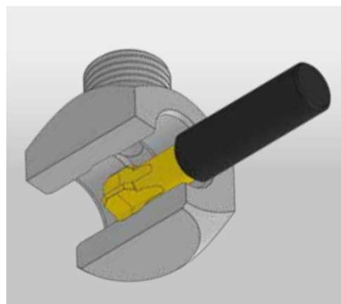
Inre konturbearbetning med Schwanog-formfräs
