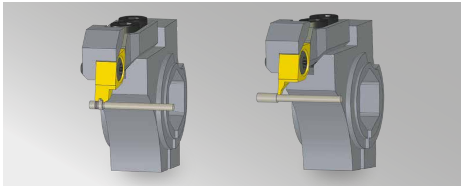
左边：成型刀片 右边：车削和扯断刀片和
