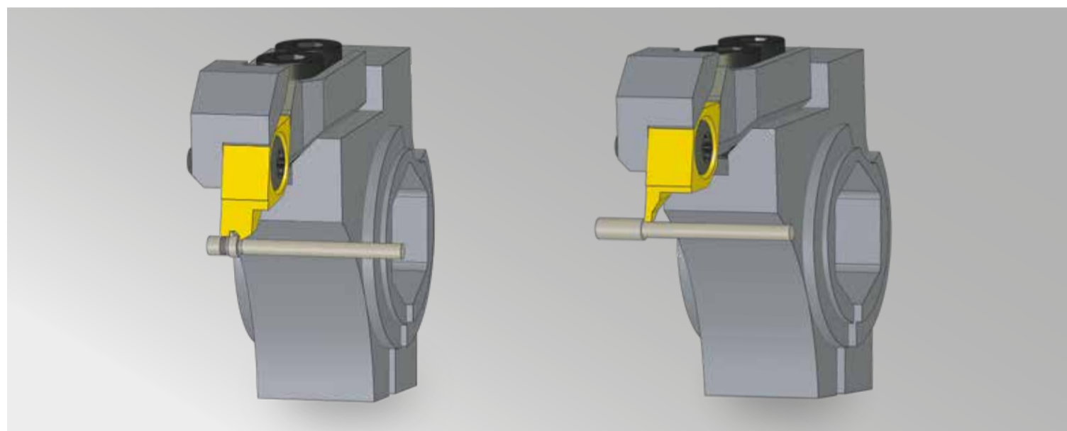
Nástroj vlevo: Tvarový zapichovací nástroj Nástroj vpravo: Kopírovací a upichovací nástroj
