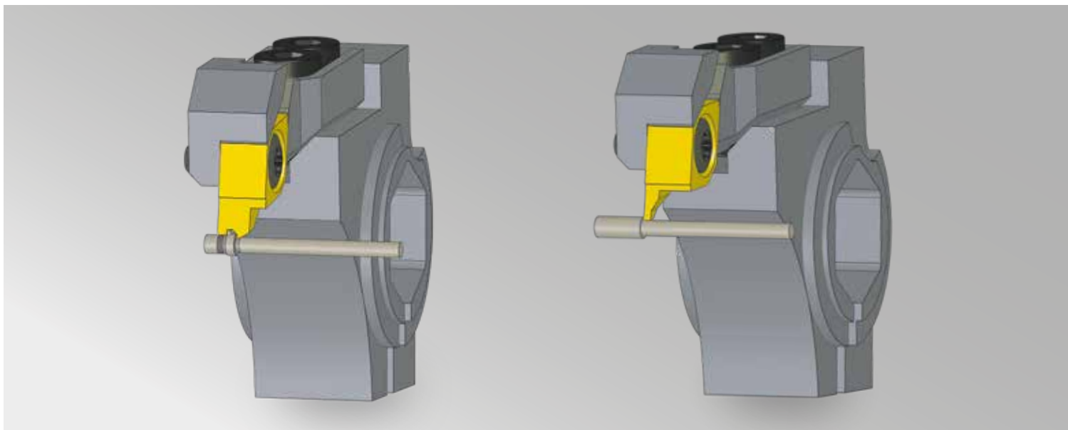
Izquierda: Herramienta de conformado con ranuras de guía, Derecha: Herramienta de copiado y tronzado
