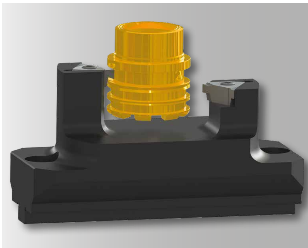
Obrábění dílu s kombinovaným držákem
