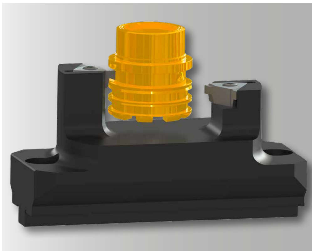
Obróbka złączki oprawką przesuwaną
