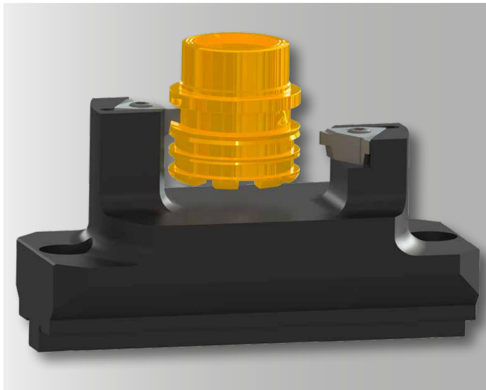
Bearbetning av anslutning med glidhållare
