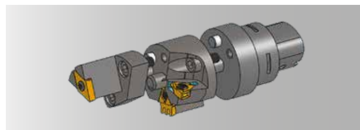
Kombinovaný nástroj HDT 2.0, modulární namontovaný systém nástrojů
