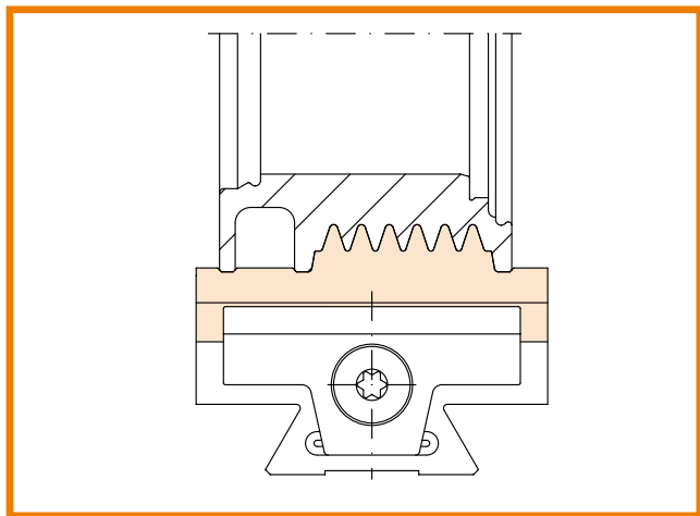
PWP-E 系统
